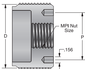
Figure 56 MPI™ Nut Die
