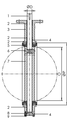
Side View Wafer & Lug Style
