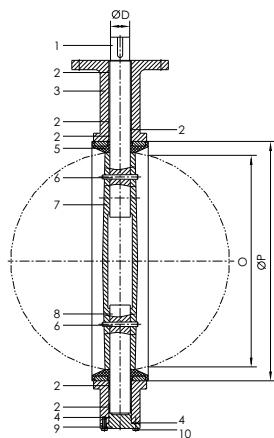
Side View Wafer & Lug Style
